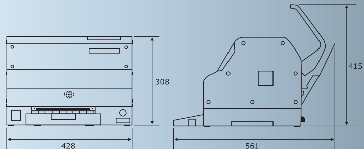
寸法 単位 [mm]
